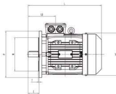
IM B5 (IM 3001) - V1 (IM 3011)
