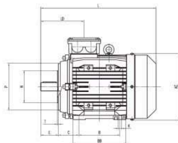
IM B35 (IM 2001)
