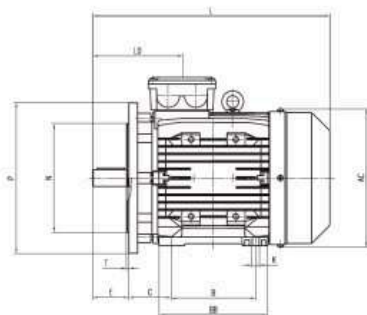
IM B35 (IM 2001)
