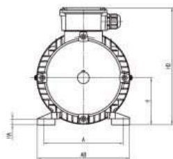
IM B3 (IM 1001)
