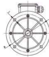
IM B5 (IM 3001) - V1 (IM 3011)
